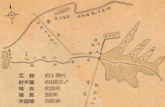
小田川ダム建設予定地略図
