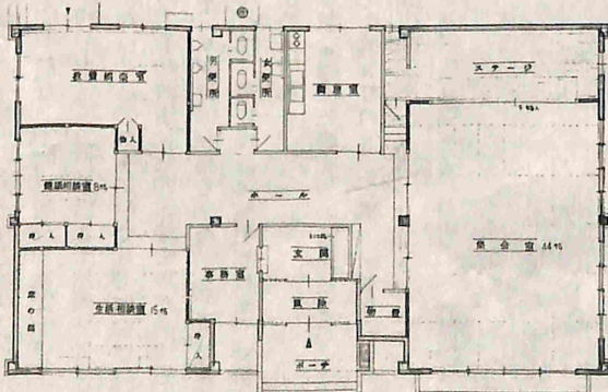
嘉瀬老人福祉センター平面図
