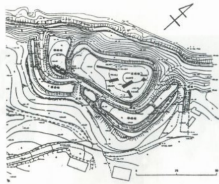
第2図 真言館跡トレンチ設定図
