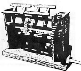
二ツ取座繰器(リヤンドリ)
