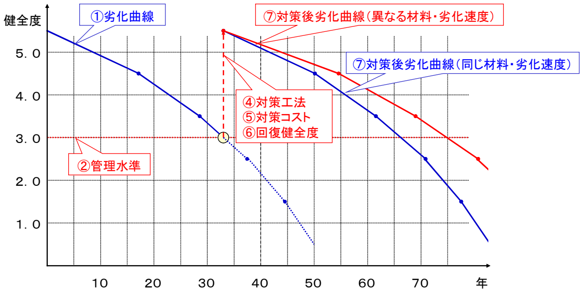
図 5-9 LCC算定
