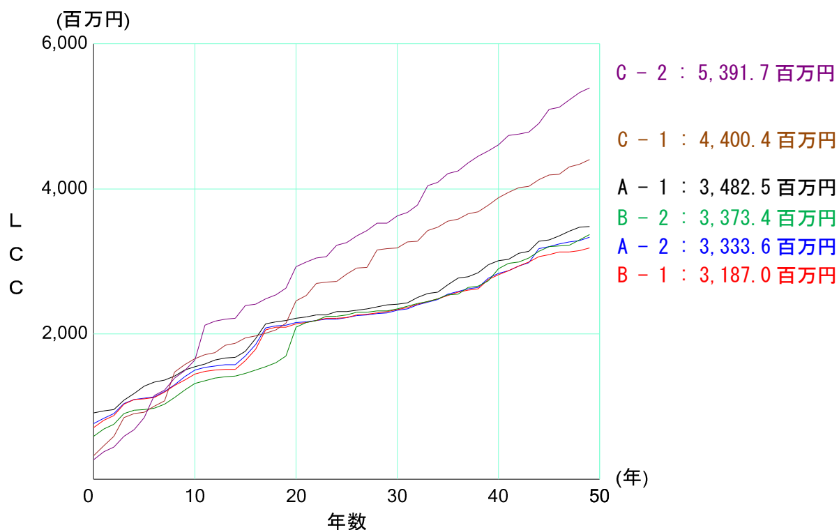
図 5-11 シナリオ別 LCC 算定結果
