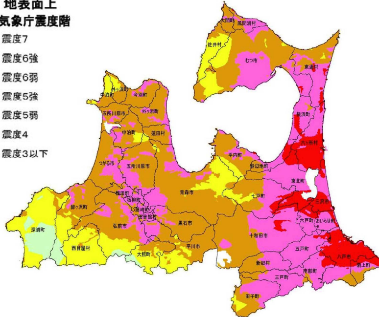
太平洋側海溝型地震の震度分布
