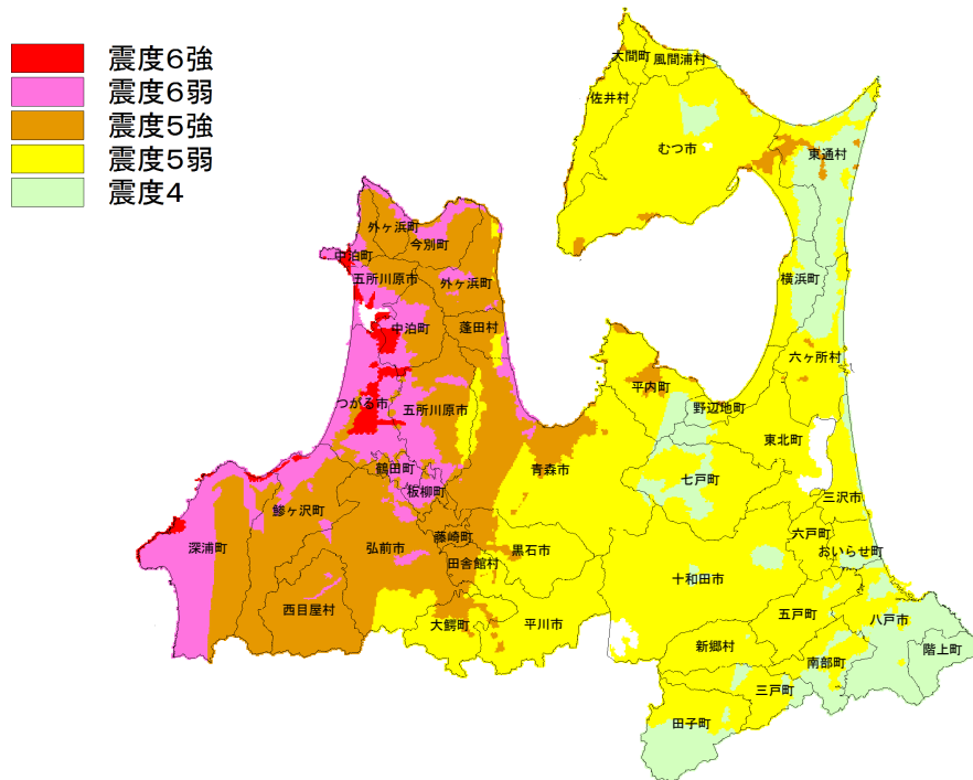
日本海側海溝型地震の震度分布
