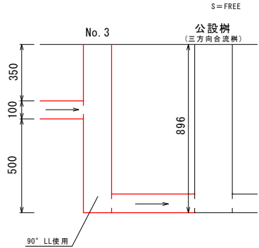
ドロップ・公設樹詳細図
