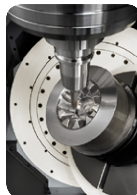
5軸MC加工機(右)
